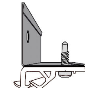
fig. 03 : Pose cornière métallique
