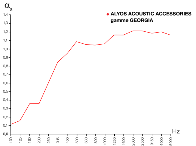
Mesure du pouvoir d'absorption du son dans une pièce réverbérante UNI EN ISO 354. Panneaux Georgia/Snowsound® installés côte à côte avec un espacement de 20 cm
